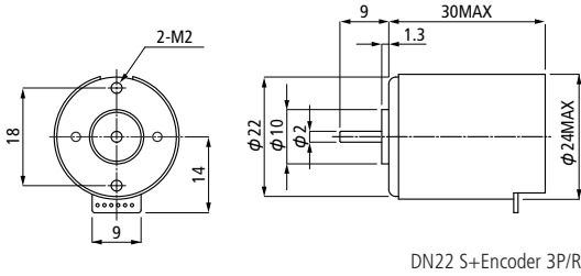
DN22 S+Encoder 3P/R
