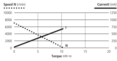
EN22 12V
