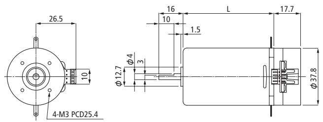
FN38+エンコーダ 200/512 P/R
