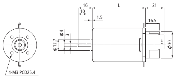
FN38+エンコーダ 60P/R
