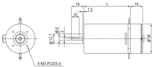
FN38+エンコーダ 1000P/R
